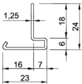
Battue de recouvrement 30011/2 0310430
